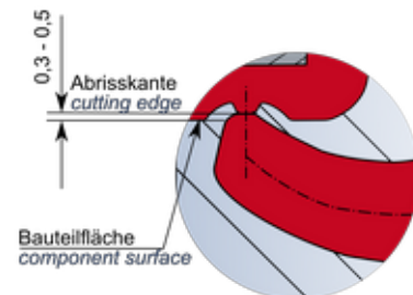
Fertige Kalottenkonstruktion Finished calotte drawing
