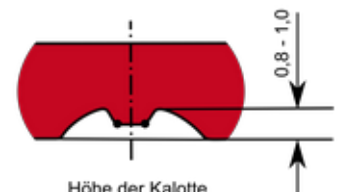
Höhe der Kalotte Height of the calotte
