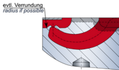
Bei Schnittpunkt Bohrung / Tunnel Winkel von 60° bis 90° festlegen Define 60 to 90 angle at bore / tunnel intersection point
