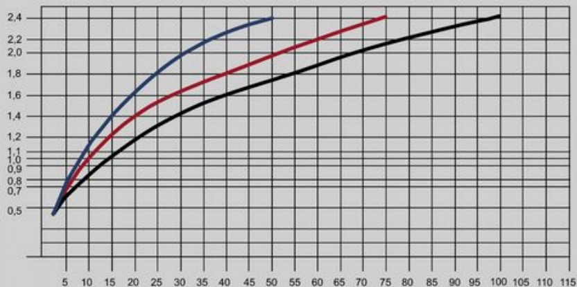
Viskositätstabelle - Table of viscosity
